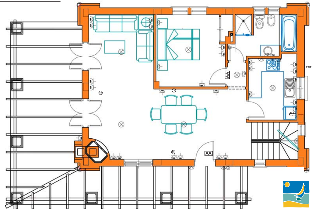
Planta Baja y Verandas / Ground Floor and Veranda
